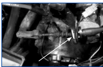
Bloccaggio del cavo della frizione
